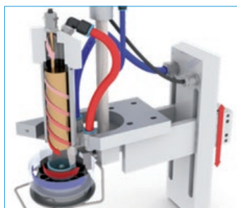
L'énergie est économisée durablement grâce à l'injection d'air comprimé froid dans la station d'air chaud
